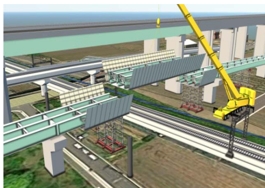
(b) トラッククレーン架設
