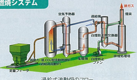
過給式流動炉のフロー
